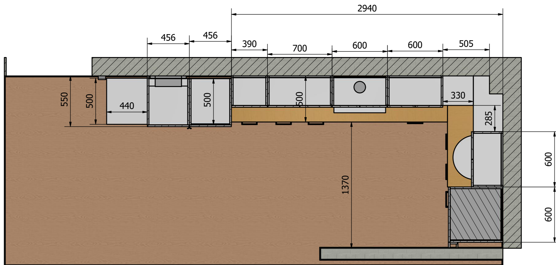
A-A ( 1 : 20 )
